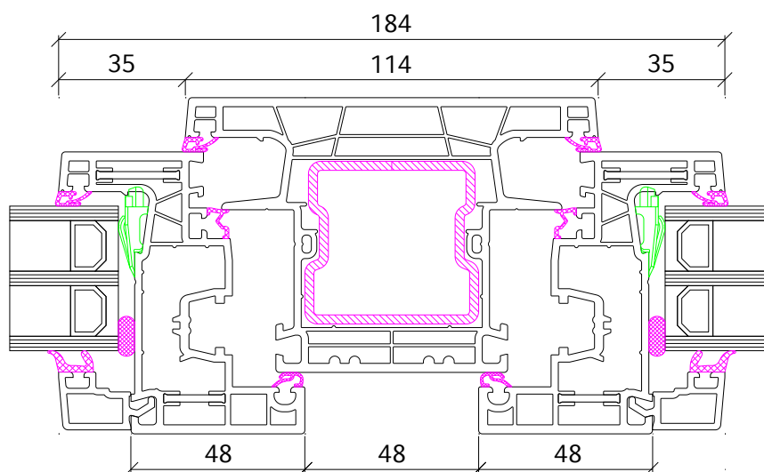
Pfosten 94 mm - Flügel 75 mm
