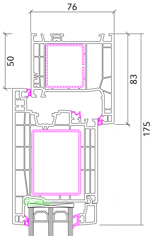
Rahmen 83 mm - Flügel 125 mm
