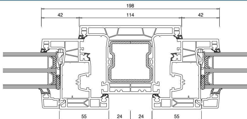
Pfosten 114 mm - Flügel 75 mm
