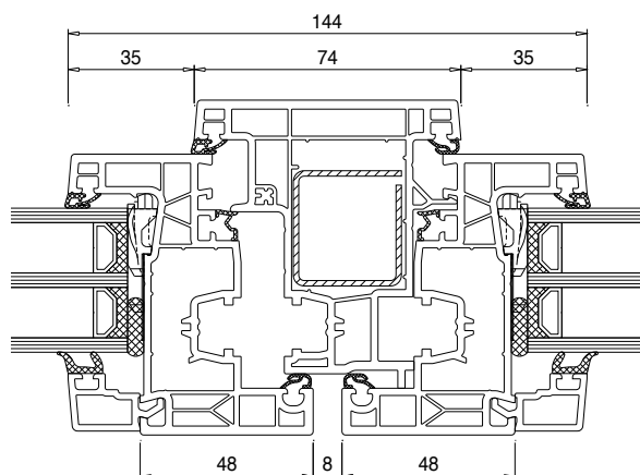
Stulp 54 mm - Flügel 75 mm
