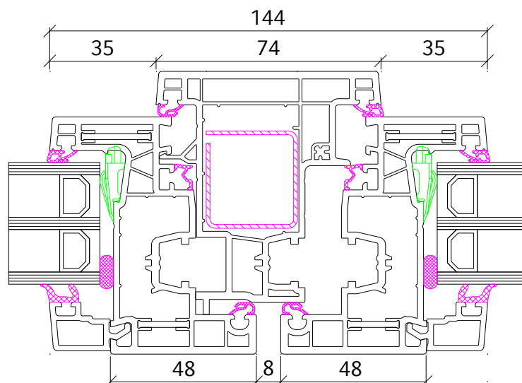
Stulp 74 mm - Flügel 68 mm
