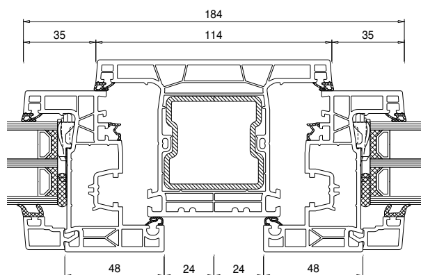
Pfosten 94 mm - Flügel 75 mm
