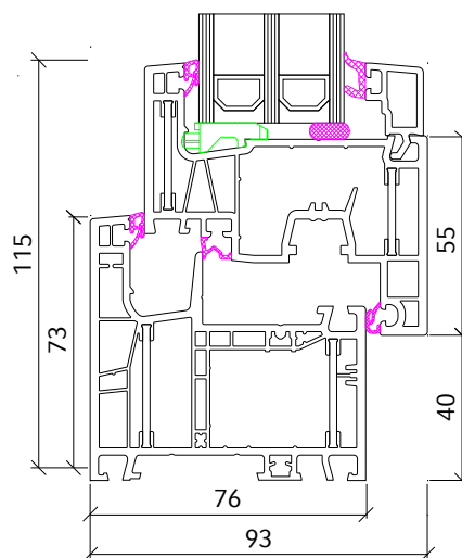
Rahmen 73 mm - Flügel 75 mm
