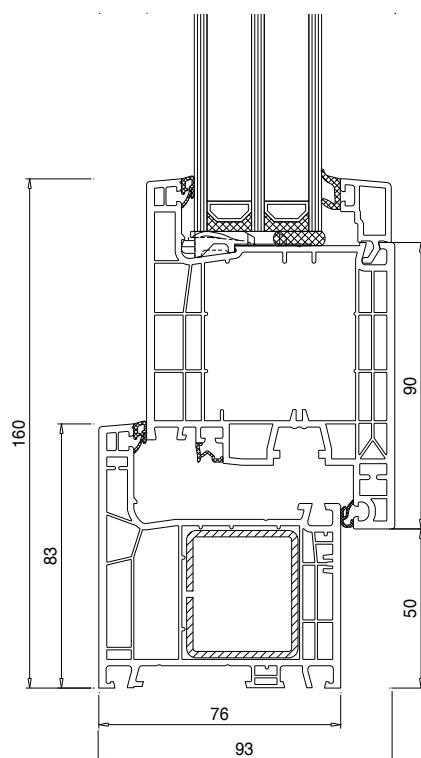
Rahmen 83 mm - Flügel 110 mm
