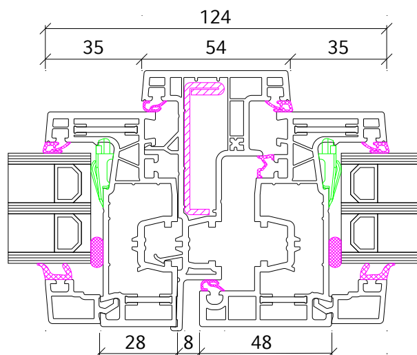
Stulp 74 mm - Flügel 68 mm
