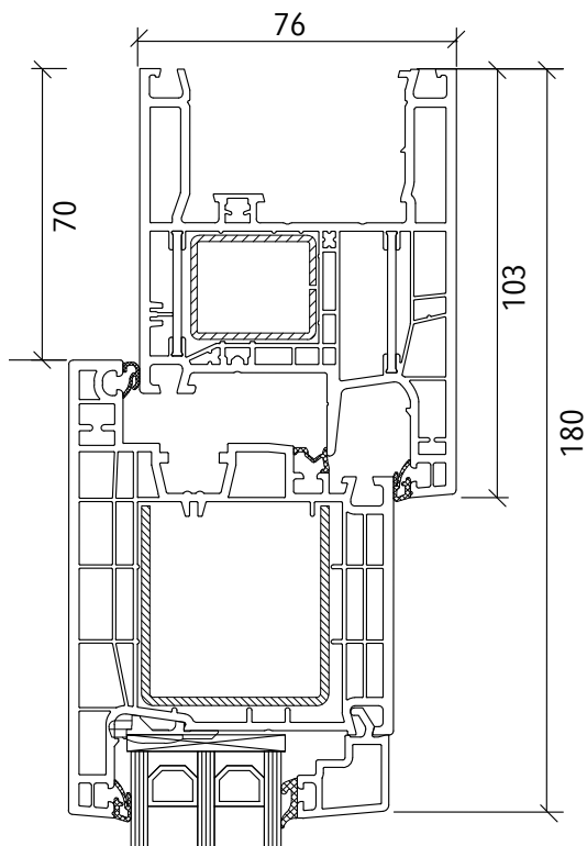
Schwelle 20 mm - Flügel 110 mm
